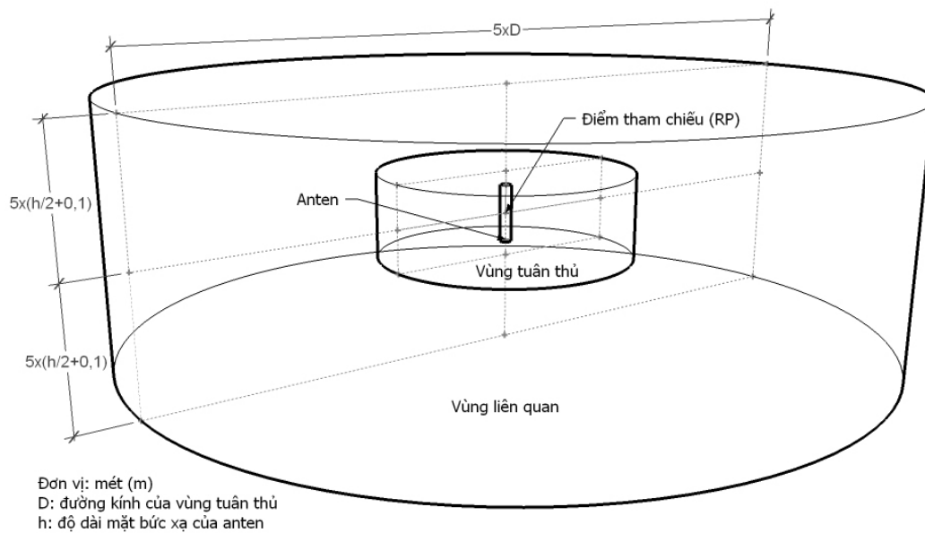
Hình 8 - Vùng liên quan của anten đẳng hướng
