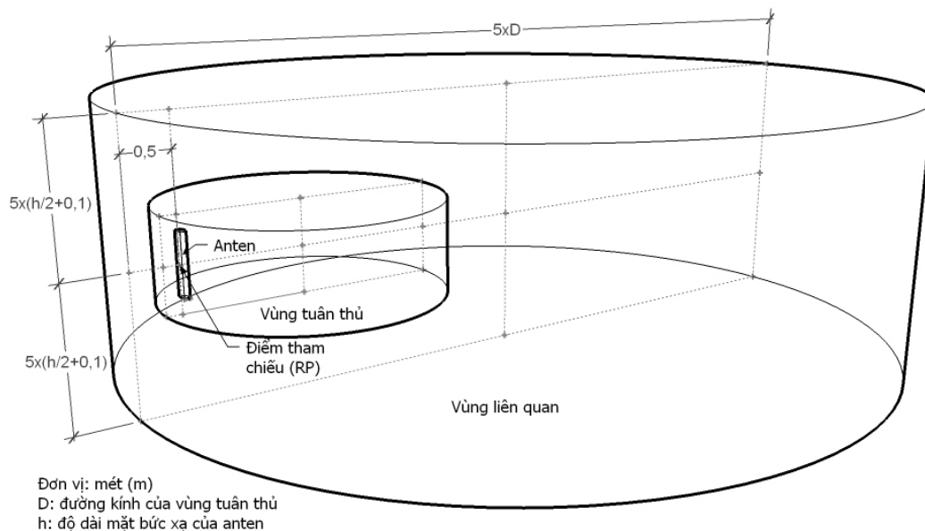
Hình 7 - Vùng liên quan của anten định hướng
